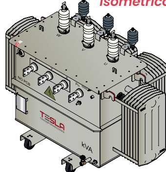
Isométrico
